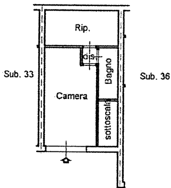
Sub. 21 PIANO SEMINTERRATO H. m. 2.40
